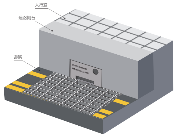
道路积水检测示意图
