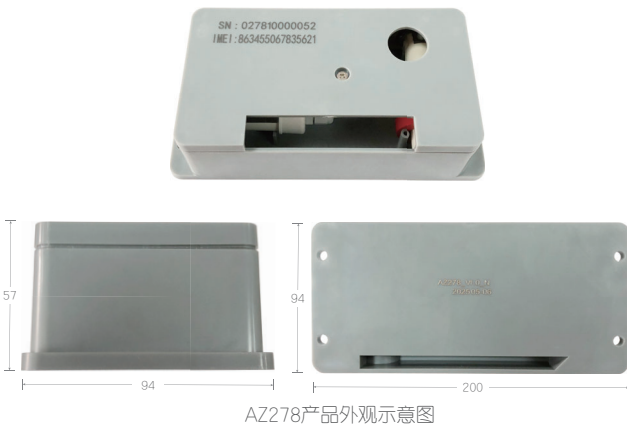
AZ278产品外观示意图
